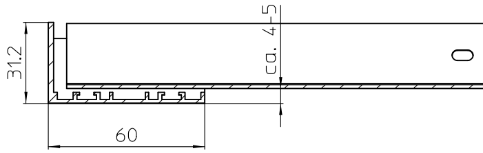
Schnitt Seitenabschluss Maßstab 1:2
